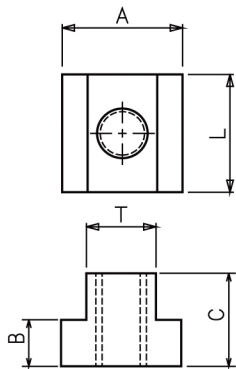
(寸法表) T・S=機械のテーブルスロット幅
